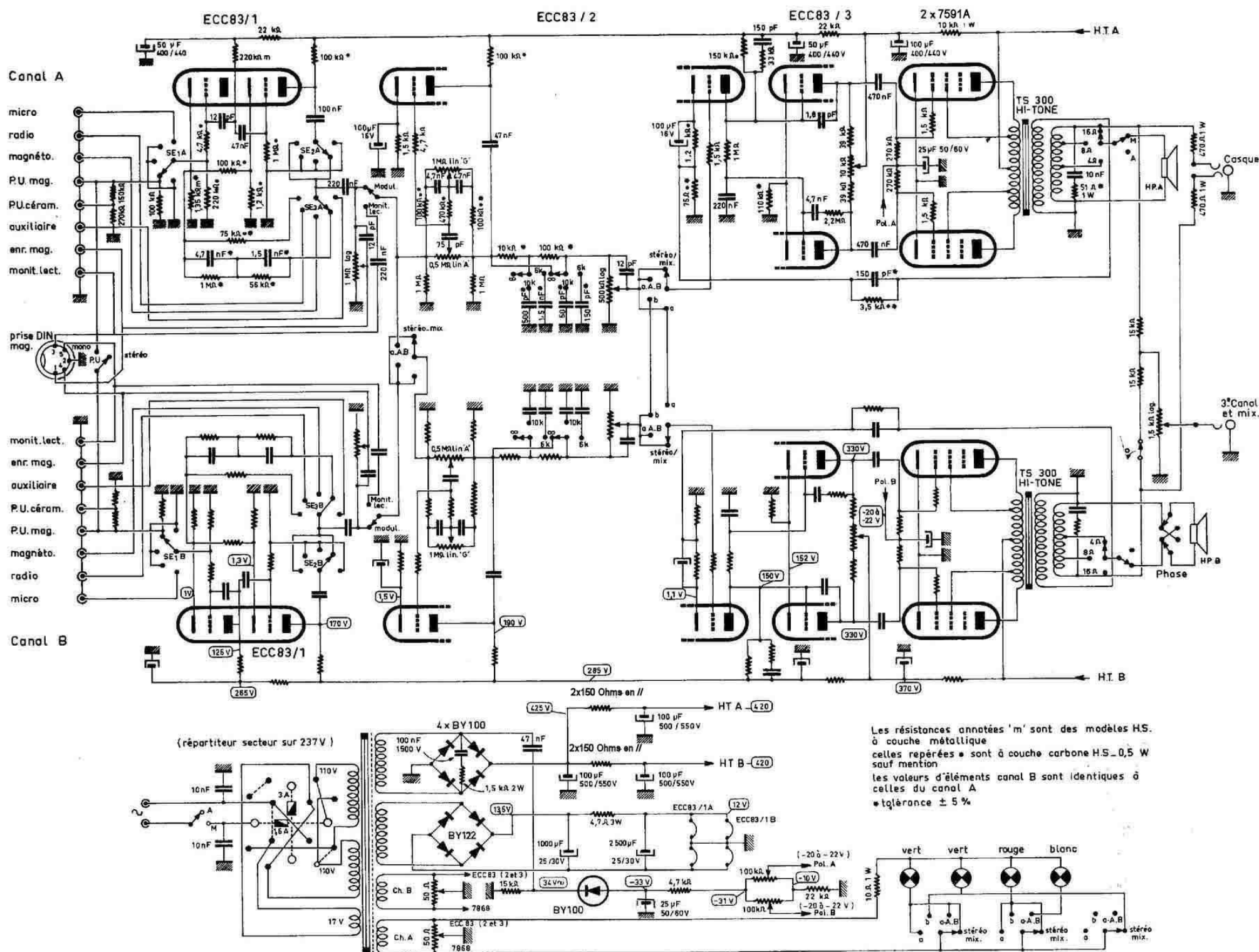
Schéma de principe de l'amplificateur H300, dont on remarquera l'étroite parenté avec celui du précédent H225.
