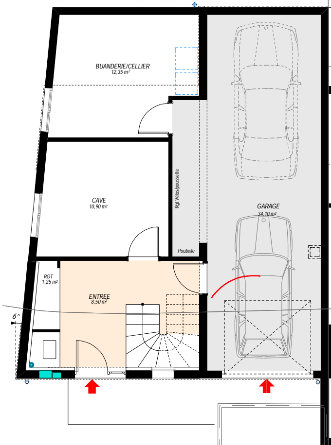
REZ DE CHAUSSEE
