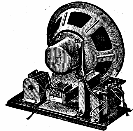
Châssis ÉLECTRODYNAMIQUE POWER-TONE
