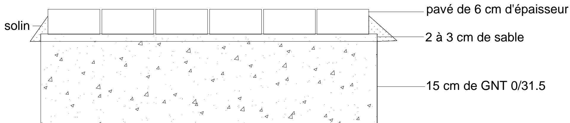
coupe technique d'une pavage carrossable
